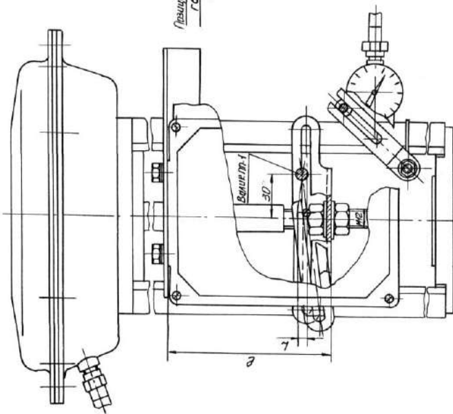
Рис. 24 Испытание - см. рис. 18
